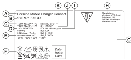
Afb. 154 Typeplaatje (voorbeeld)
