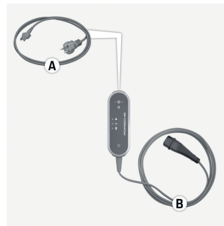
Obr. 266 Přípojky na řídicí jednotce
