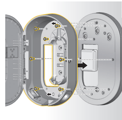
Billede 211 Skru ladedock fast på monteringsplade
