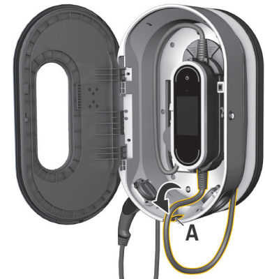
Billede 217 Montering af betjeningsenhed
