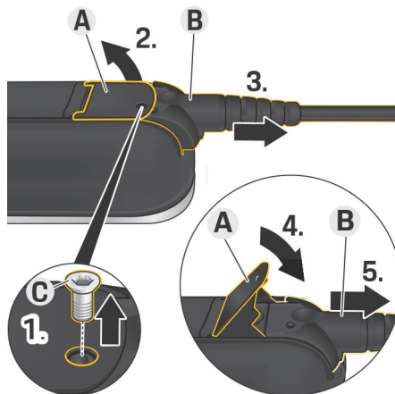
Obr. 389 Odpájanie káblov
