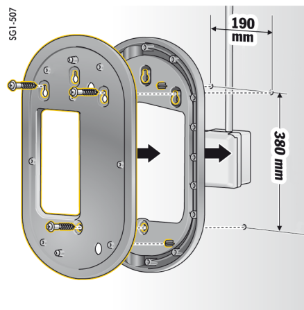
298. ábra Fúrási méretek
