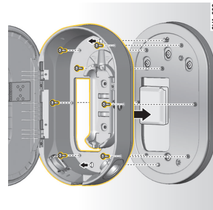
Obr. 387 Zaskrutkovanie nabíjacieho doku do montážnej dosky
