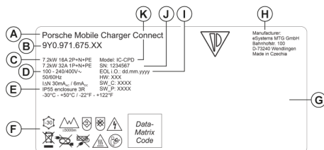
Obr. 396 Typový štítok (príklad)
