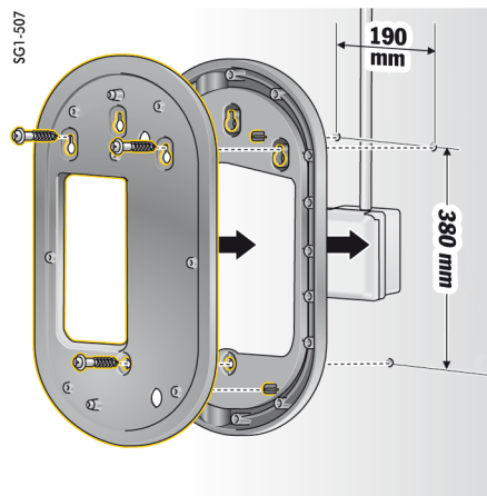
Billede 210 Boreskabelon
