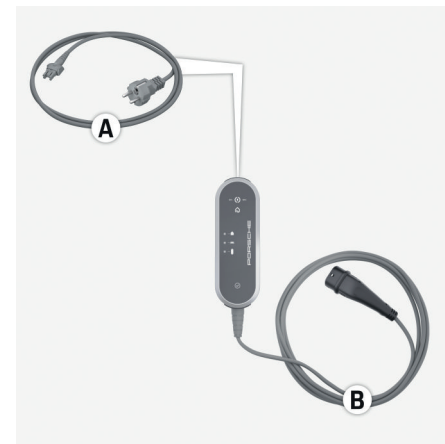
Billede 200 Tilslutninger på betjeningsenheden
