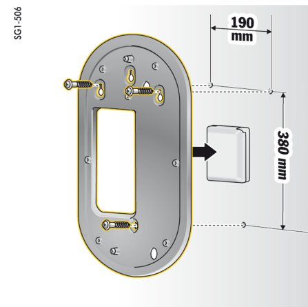
Kuva 186 Porausmitat
