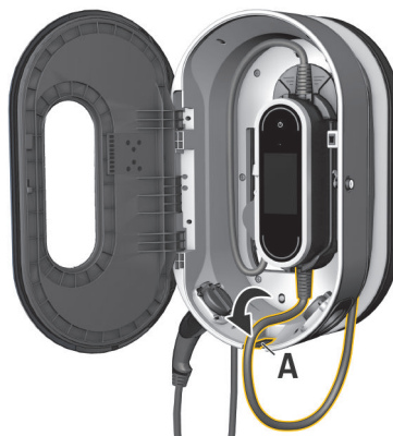
Afb. 151 Bedieningseenheid ophangen
