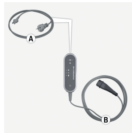
Fig. 90 Conexiones en la unidad de control
