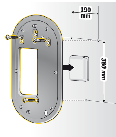
Фиг. 516 Размери за пробиване
