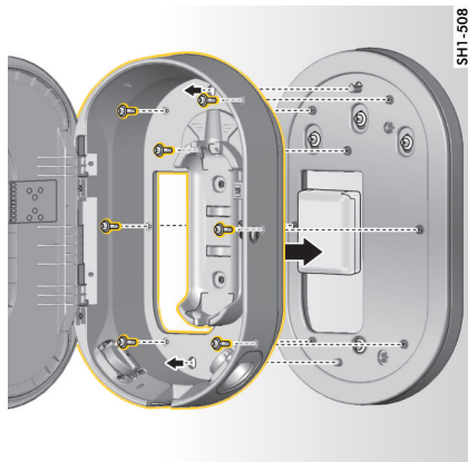
Billede 209 Skru ladedock fast på monteringsplade
