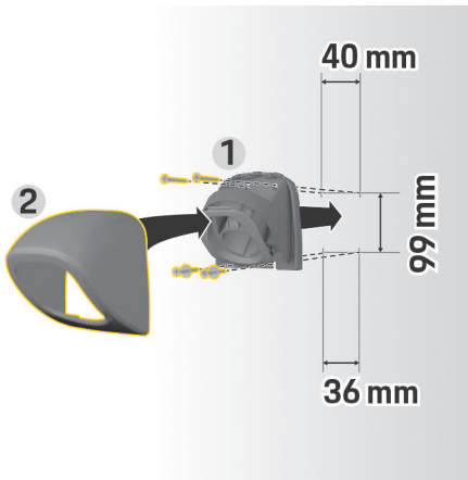
Joonis 426 mõõtmed puurimiseks
