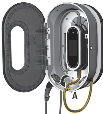
305. ábra A kezelőegység rögzítése
