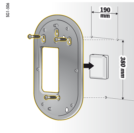
Rys. 318 Wymiary otworów
