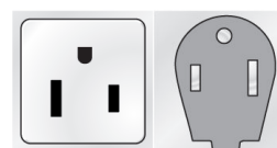
NEMA 6-50 Dåse/stik
