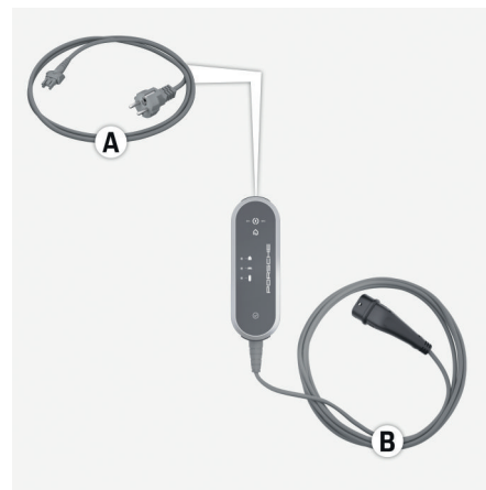
Bild 156 Anslutningar på manöverenheten
