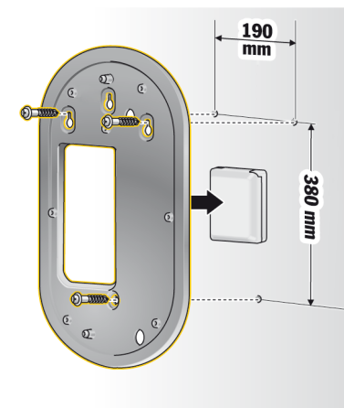
Obr. 274 Schéma vrtání
