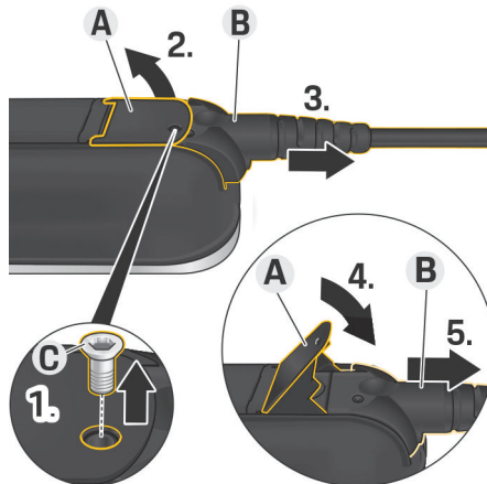
Rys. 323 Odlączenie kabla
