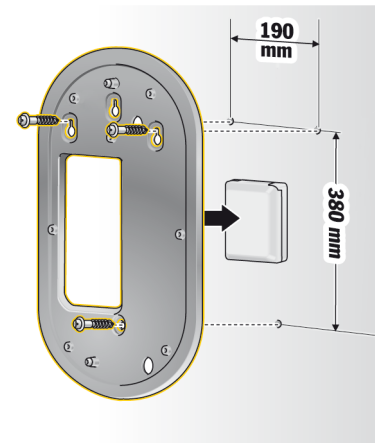
Fig. 494 Dimensiuni de găurire
