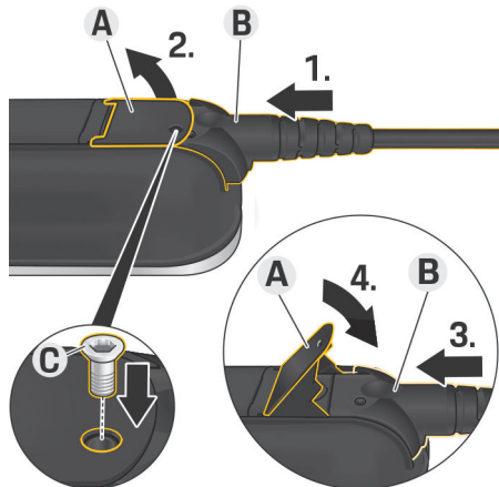
Billede 214 Fastgør kablet, og fikser stikket
