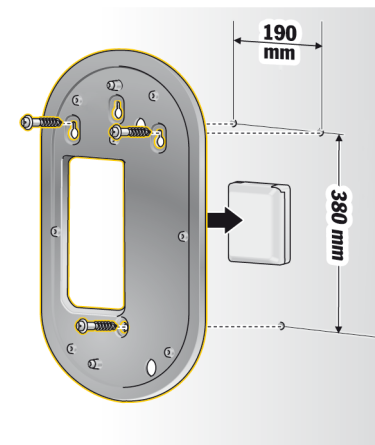
Fig. 230 Bormål
