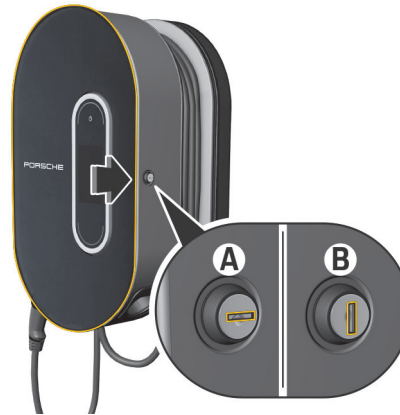
Billede 216 Ladedock
