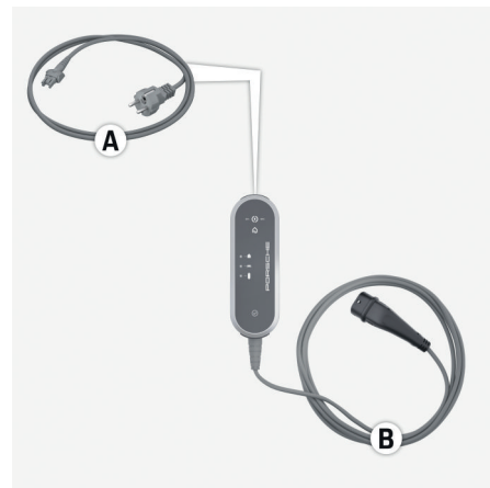
442 pav. Valdymo bloko jungtys
