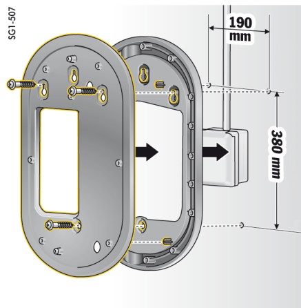
Sl. 342 Mjere za bušenje
