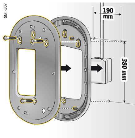
SI. 408 Mere za izvrtine
