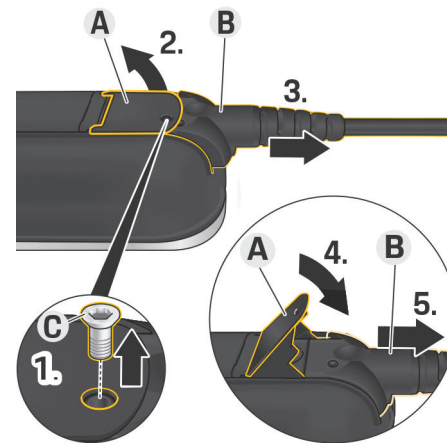
Bild 169 Lossa kabeln
