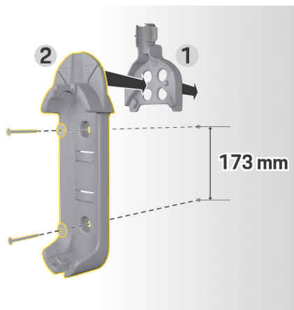
Rys. 314 Wymiary otworów
