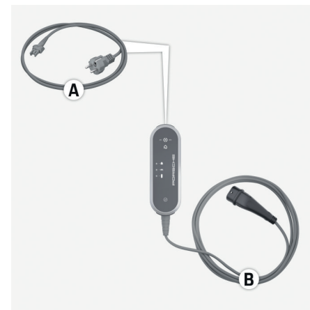
Fig. 112 Ligações na unidade de comando
