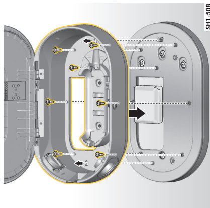
297. ábra A felszerelési lap rácsavazása a falitartóra
