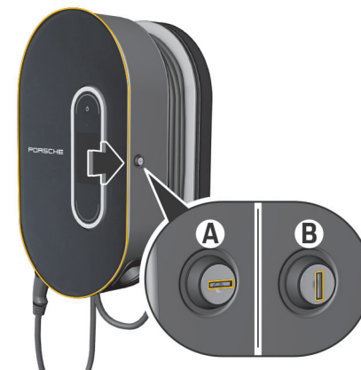
Rys. 326 Stacja ładowająca
