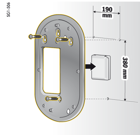
Fig. 120 Dimensões de perfuração
