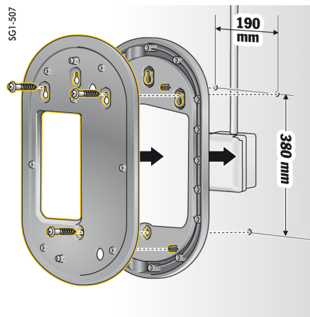
Fig. 122 Dimensões de perfuração
