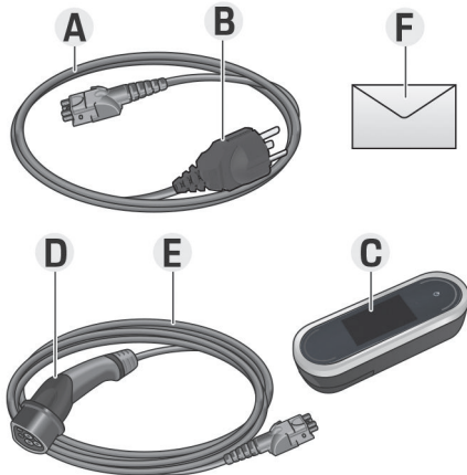
Obr. 375 Rozsah napájania
