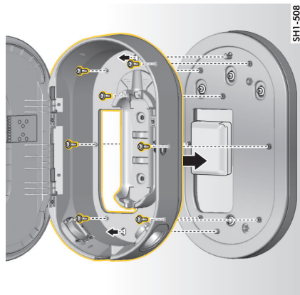
Abb. 11 Lade-Dock an Montageplatte schrauben
