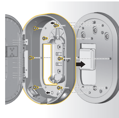
299. ábra A felszerelési lap rácsavazása a falitartóra
