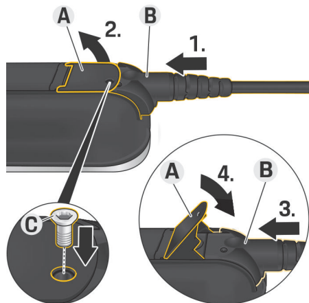
Sl. 346 Pričvršćivanje kabela i fiksiranje utikača
