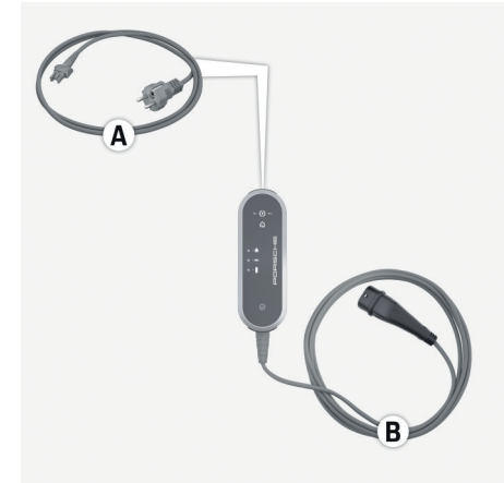
Sl. 354 Priključci na kontrolnoj jedinici
