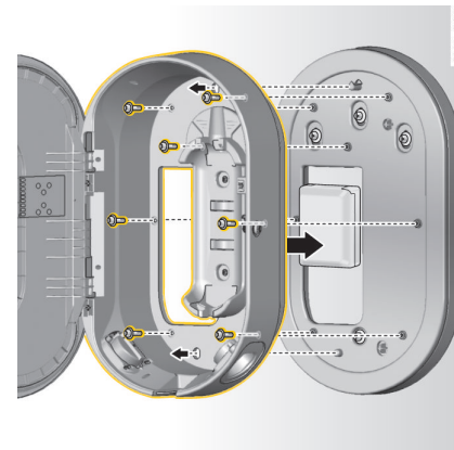
Att. 475 Uzlādes doka pieskrūvēšana pie montāžas plāksnes
