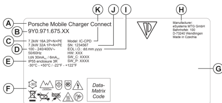
Abb. 22 Typenschild (Beispiel)
