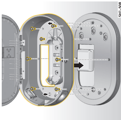
SI. 407 Pritrditev polnilne postaje na montažno ploščo
