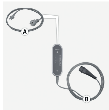
Fig. 486 Conexiunile de pe unitatea de control
