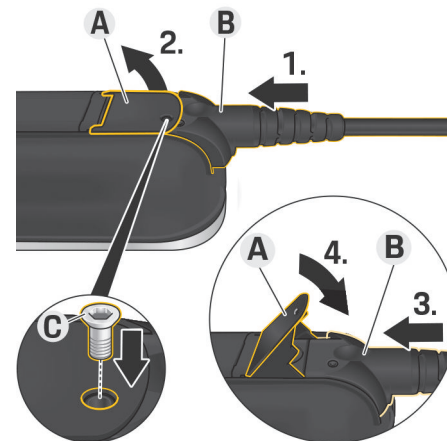
Εικ. 258 Σύνδεση καλωδίων και στερέωση ρευματοληπτών
