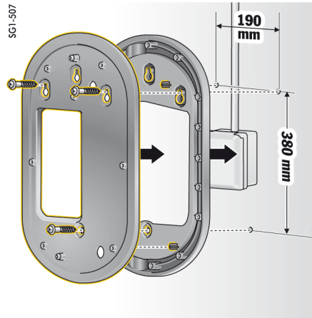
Fig. 496 Dimensiuni de găurire
