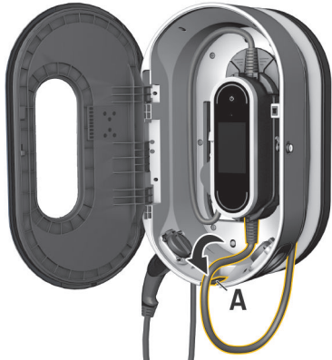
Kuva 195 Käyttöyksikön kiinnittäminen
