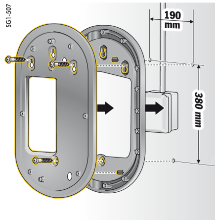
Joonis 430 Mõõdud puurimiseks
