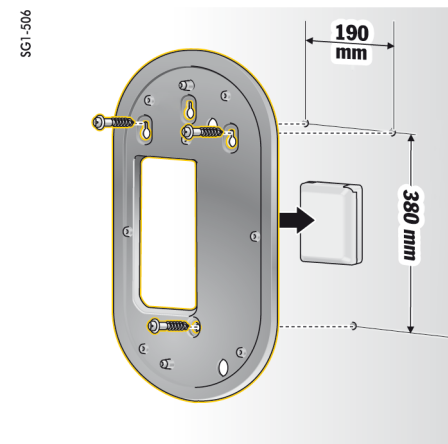
Obr. 384 Rozmery otvorov
